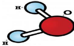
تصویر (۳۱): شکل مولکول آب.
