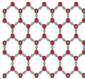
تصویر (۳۲): این تصویر به روشنی نشان می‌دهد که اتم‌های آب به شکل شش ضلعی کنار یکدیگر مرتب شده‌اند.
