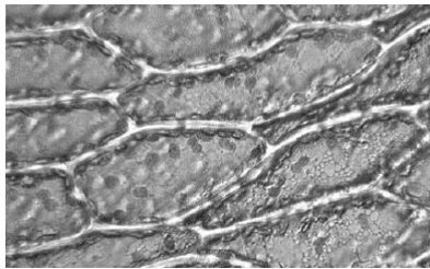
تصویر (۳۸): شکل شش‌ضلعی سلول‌های گیاهی.
