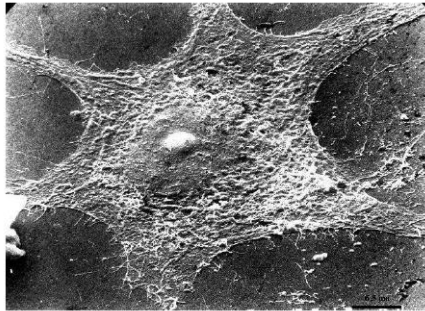
Une Cellule en Culture, vue au Microscopie Electronique à Balayage (M.E.B.) (c) Copyright - U.F.R.-S.V.E. - C.M.E.B. - 1997
